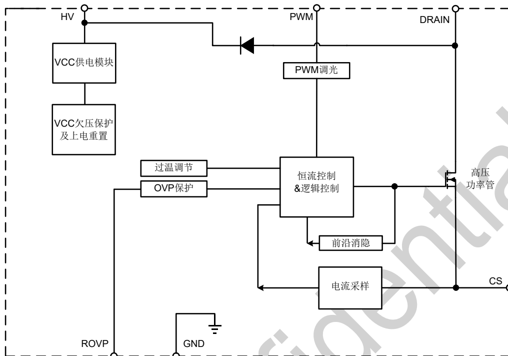
图 3 BP2956XD 内部框图
