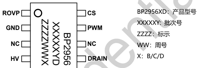
图 2 管脚封装图
