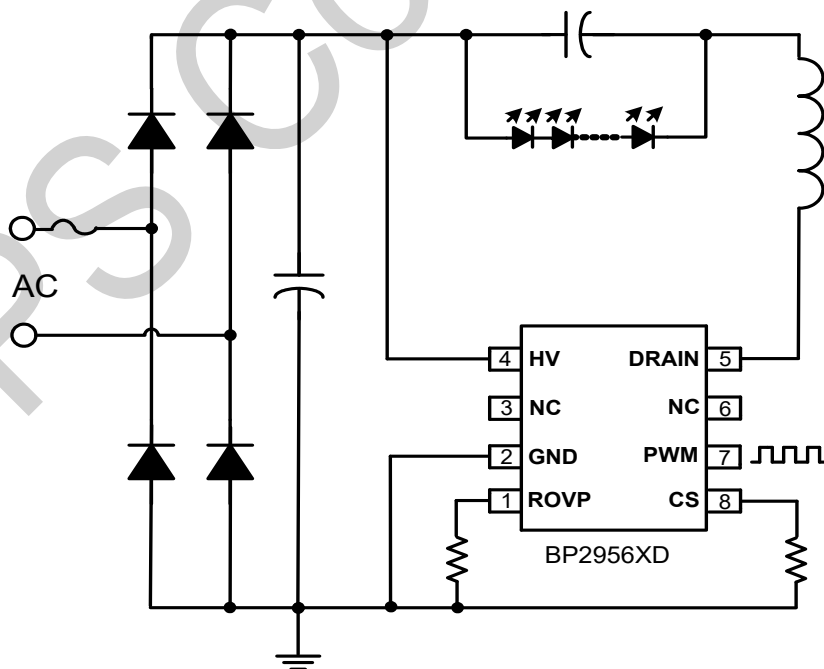
图 1 BP2956XD 典型应用图
