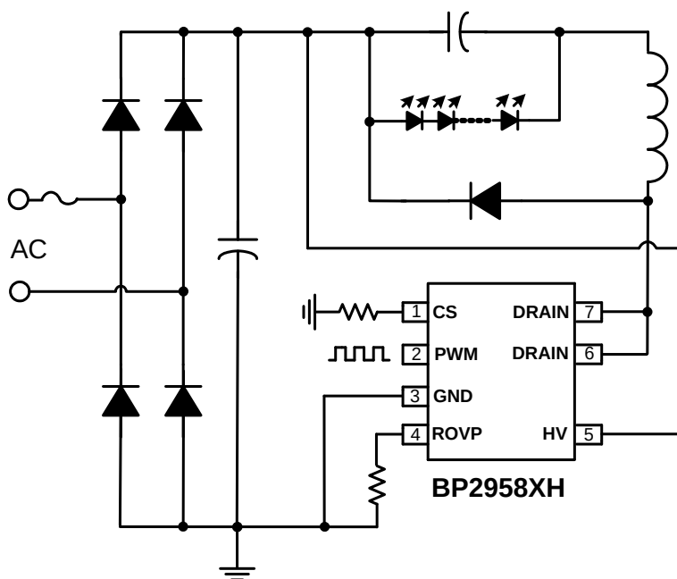
图 1 BP2958XH 典型应用图
