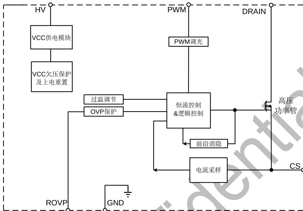
图 3 BP2958XH 内部框图
