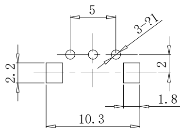
安装孔位图
