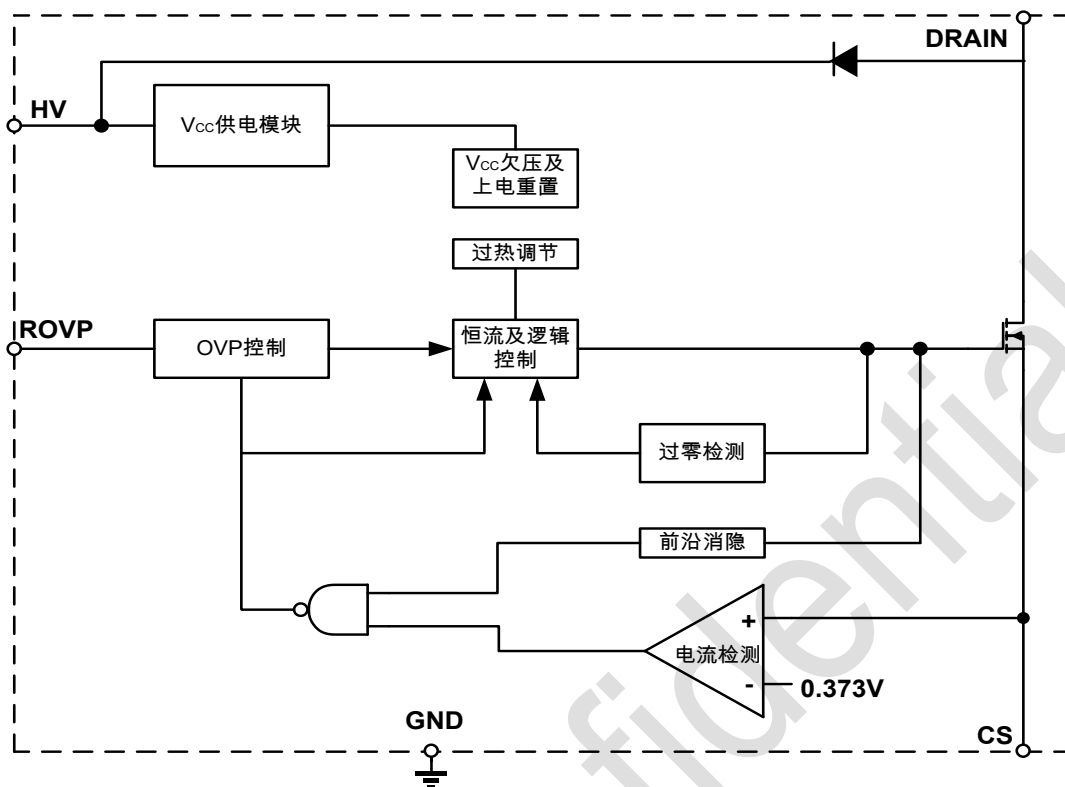
图 3 BP2861XJL 内部框图
