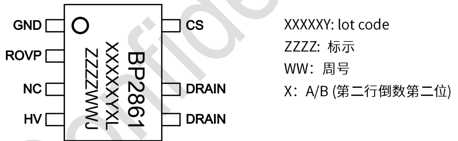
图 2 管脚封装图
