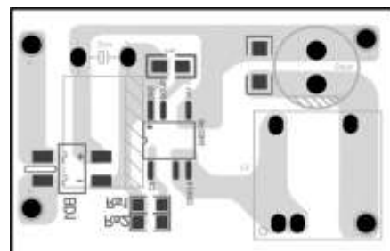
图 4 PCB 铺铜面积优化图
