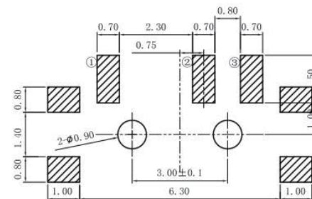
PCB安装位
