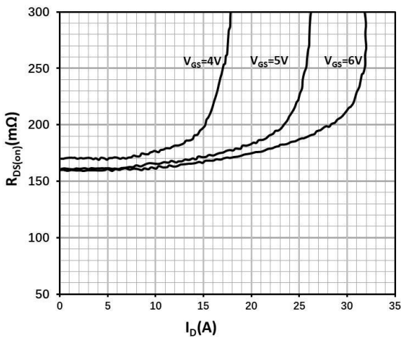
典型漏源级导通内阻曲线
