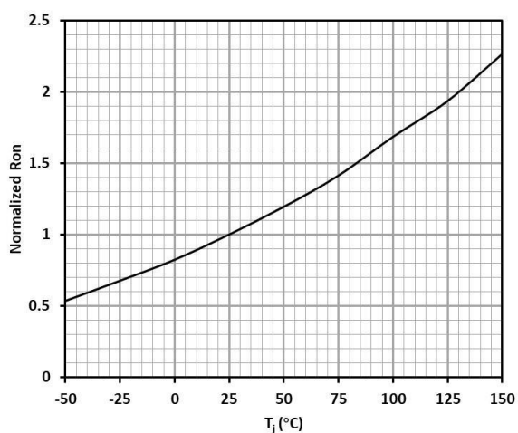
漏源级导通内阻- T_J 曲线
