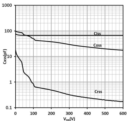
典型电容值- V_{DS} 曲线
