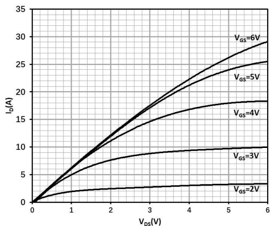
典型输出特性曲线
