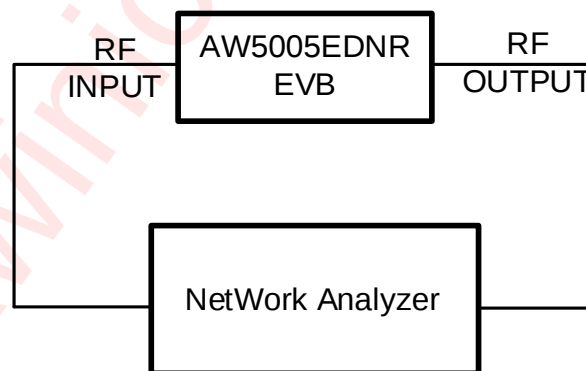
Figure 5 S Parameter Test
