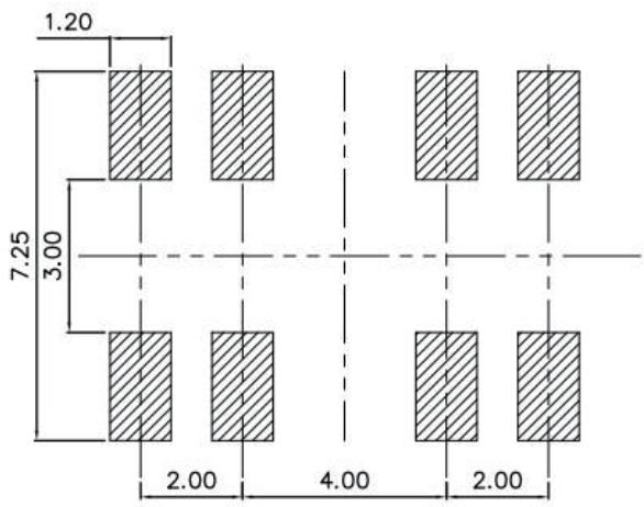
PCB安装图
