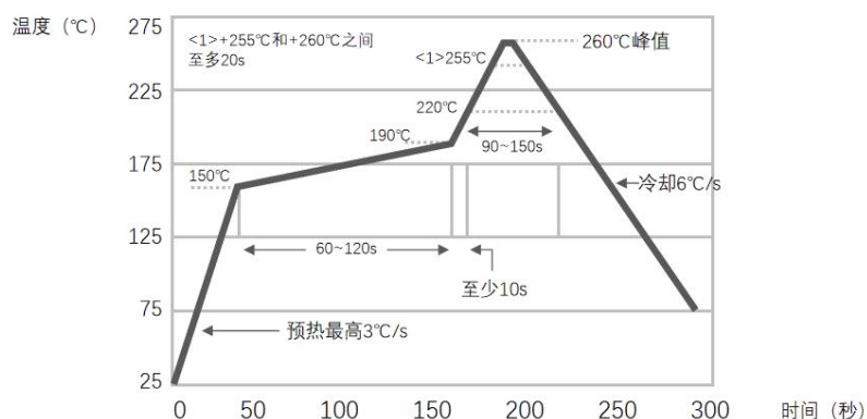
回流焊曲线图
