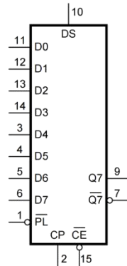
图 1 逻辑符号
