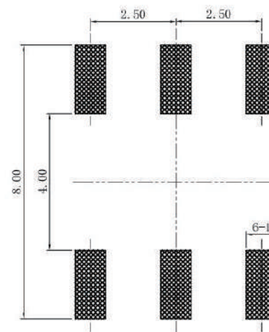
PCB安装图
