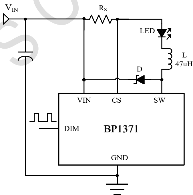
图 1 BP1371 典型应用图
