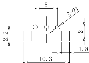
安装孔位图
