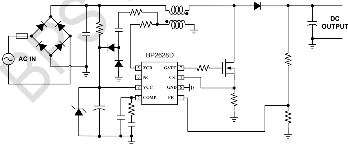
图 1 BP2628D 典型应用电路
