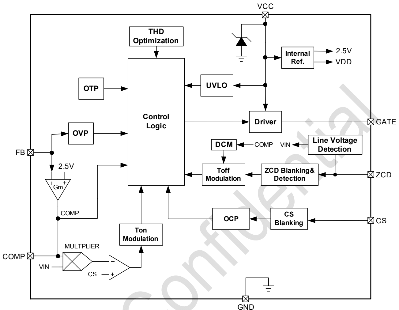
图 3 BP2628D 内部框图
