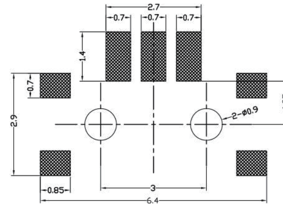
PCB安装图
