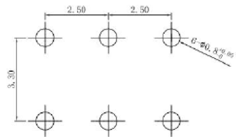
PCB安装图
