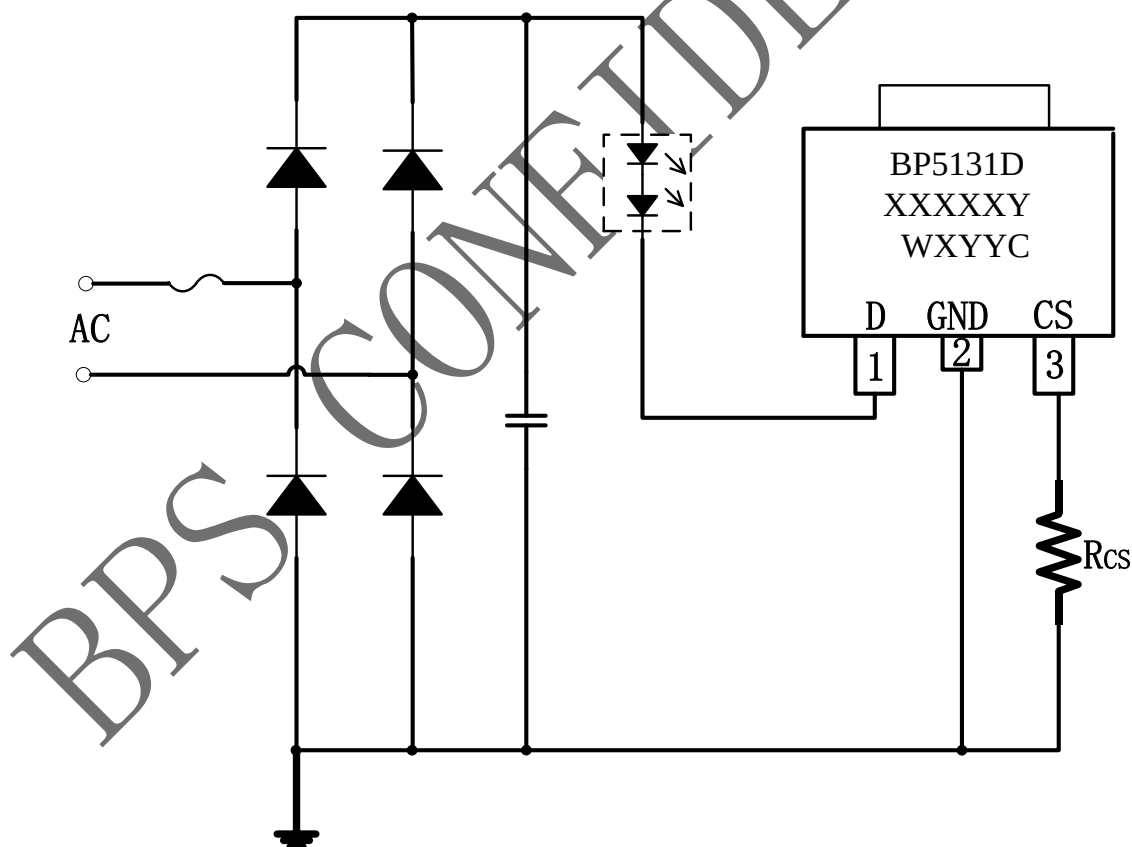
图 1 BP5131DC 典型应用图
