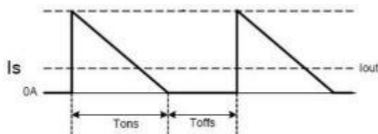
次边的电流波形
