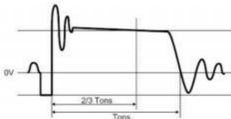
辅助端电压波形
