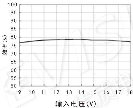
效率Vs输入电压(满载) WRF1205S-3WR2
