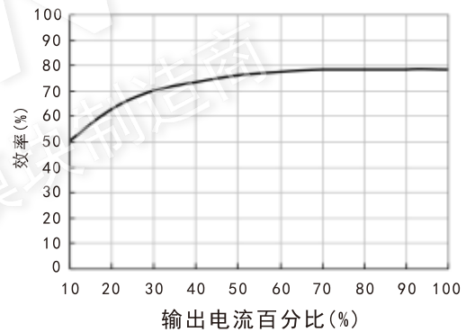
效率Vs输出负载 (Vin=12V) WRF1205S-3WR2
