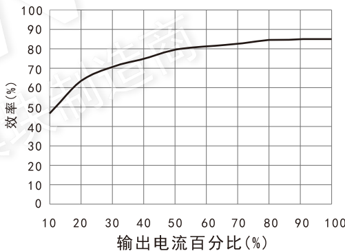
效率Vs输出负载 (Vin=24V) WRA2415S-3WR2
