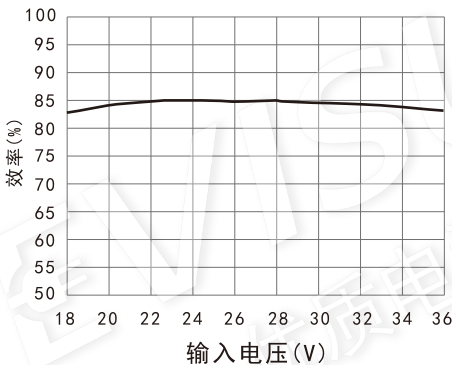
效率Vs输入电压(满载) WRA2415S-3WR2
