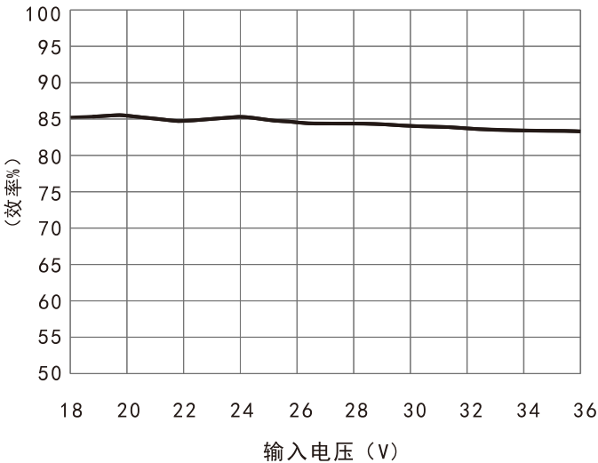
效率VS输入电压曲线图（满载）
