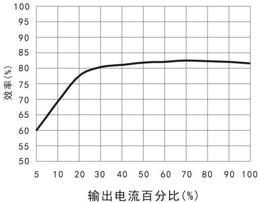
效率Vs输出负载( V_{in}=12V ) VRA1205YMD-6WR3
