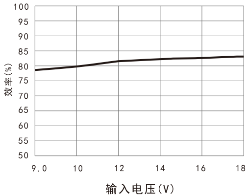
效率Vs输入电压(满载) VRA1205YMD-6WR3
