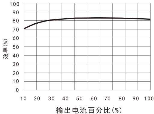
效率Vs输出负载( V_{in}=5V ) VRA0505YMD-6WR3
