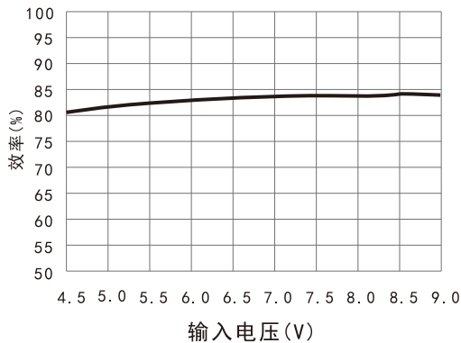
效率Vs输入电压(满载) VRA0505YMD-6WR3
