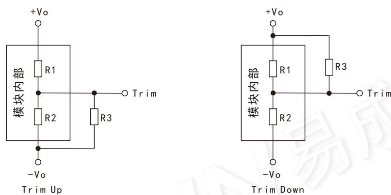
Trim使用电路（框内为模块内部电路）
