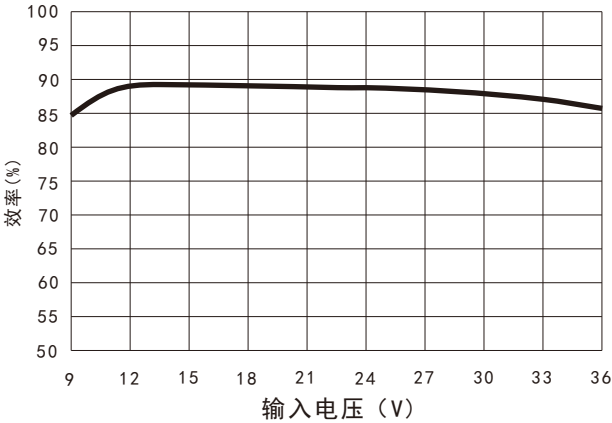
效率VS输入电压曲线图 (满载) URA2405S-10WR3
