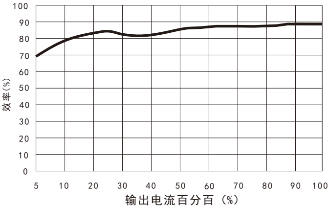
效率VS输出负载曲线图 (Vin=24V) URA2405S-10WR3
