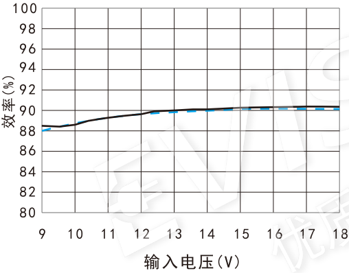
效率Vs输入电压(满载) -- VRB1205YMD-20WR3 -- VRB1212YMD-20WR3
