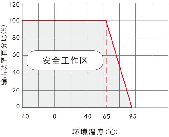
VRB24 (48)_YMD-20WR3系列 标称电压输入，3.3V、5V输出 温度降额曲线图
