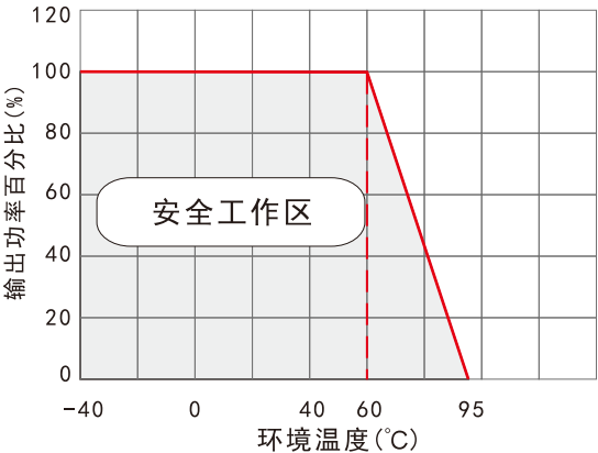
VRB12_YMD-20WR3系列 标称电压输入, 3.3V、5V输出 温度降额曲线图
