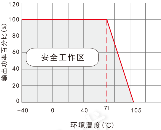
VRB24 (48)_YMD-20WR3系列 标称电压输入，其他电压输出 温度降额曲线图
