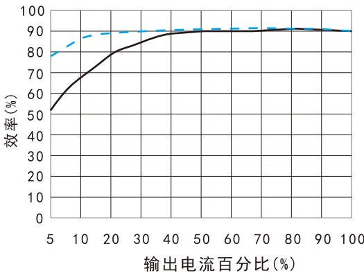
效率Vs输出负载 (Vin=24V) -- VRB2405YMD-20WR3 -- VRB2415YMD-20WR3
