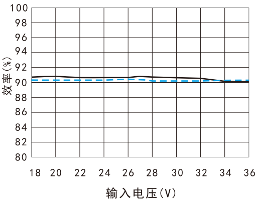
效率Vs输入电压(满载) -- VRB2405YMD-20WR3 -- VRB2415YMD-20WR3
