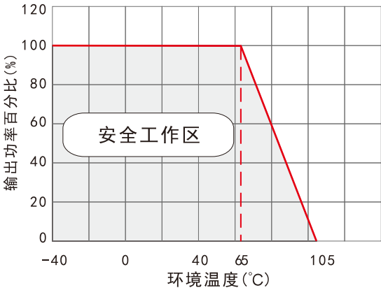
VRB12_YMD-20WR3系列 标称电压输入, 其他电压输出 温度降额曲线图
