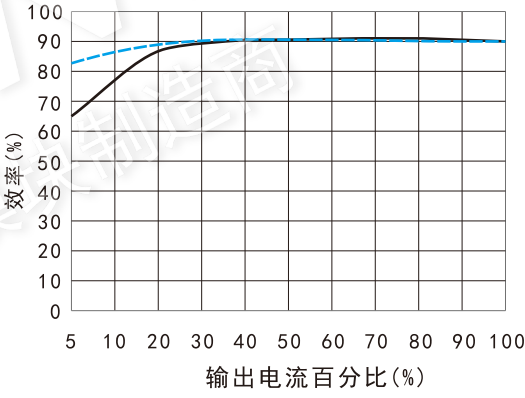
效率Vs输出负载 (Vin=12V) -- VRB1205YMD-20WR3 -- VRB1212YMD-20WR3
