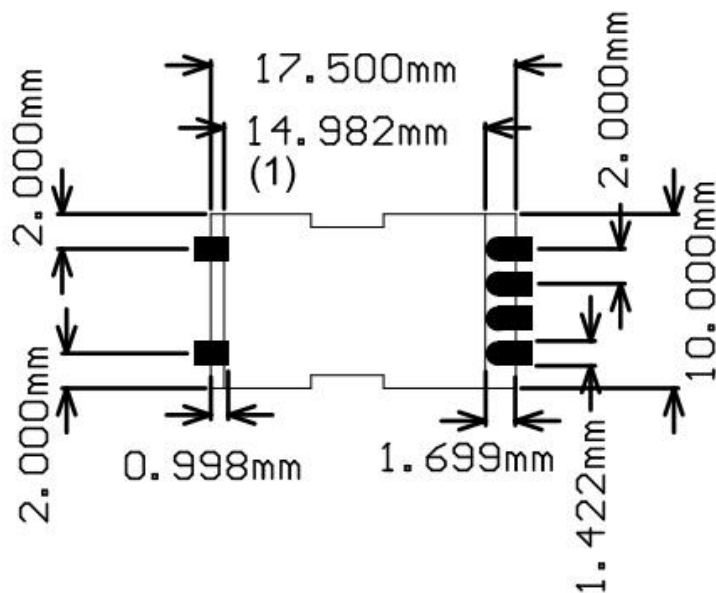
俯视图
