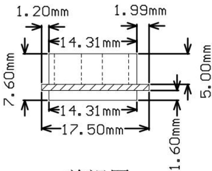
前视图
