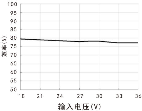
效率Vs输入电压(满载) WRB2405S-1WR2
