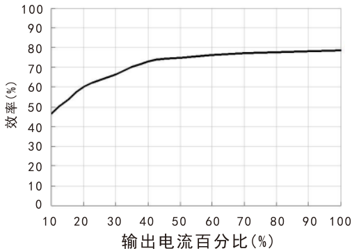
效率Vs输出负载(Vin=24V) WRB2405S-1WR2
