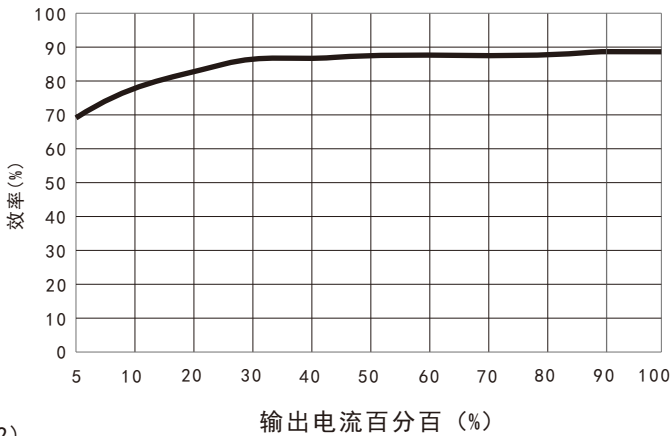
效率VS输出负载曲线图 (Vin=24V)
