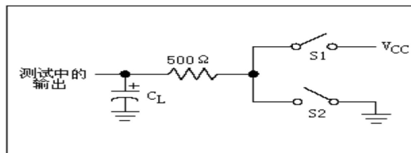
图 5:驱动器使能/无效定时测试负载
