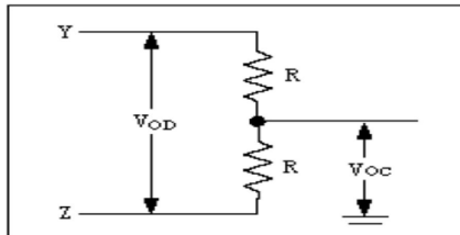
图 2:驱动器 DC 测试负载
