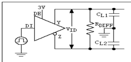
图 4:驱动器定时测试负载
