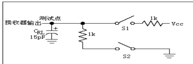
图 3:接收器使能/无效定时测试负载
