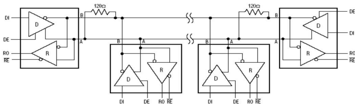
图13: 典型半双工RS-485网络
