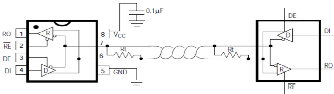
图 1：SP485EEP-TD 典型半双工应用电路
