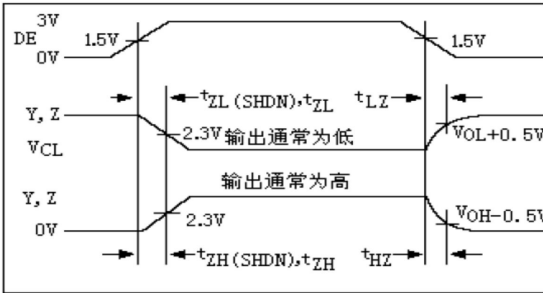
图 7:驱动器使能和无效时间
