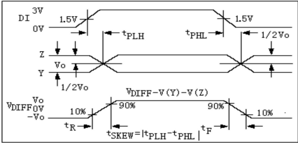
图 6:驱动器传播延时
