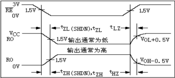
图 9:接收器使能和无效时间
