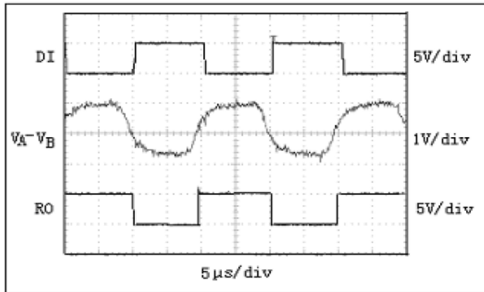
图 12: 在 50kHz 时驱动 4000 英尺的电缆
