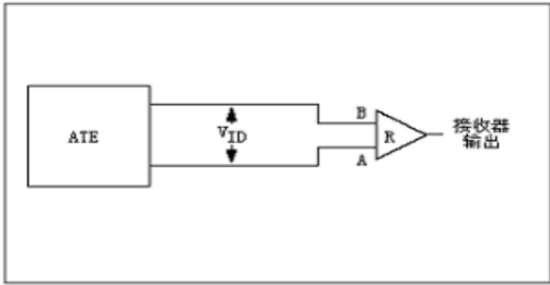
图 10:接收器传播延时测试电路
