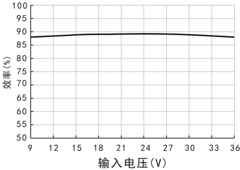
效率Vs输入电压 (满载) URB2405LD-20WR3
