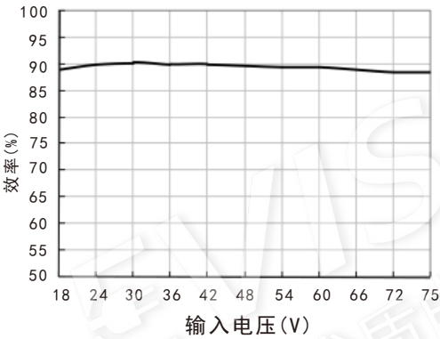
效率Vs输入电压 (满载) URB2405LD-20WR3
