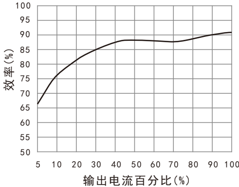
效率Vs输出负载( V_{in}=48\text{V} ) URF4815P-6WR3
