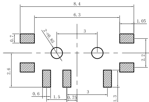
安装参考图
