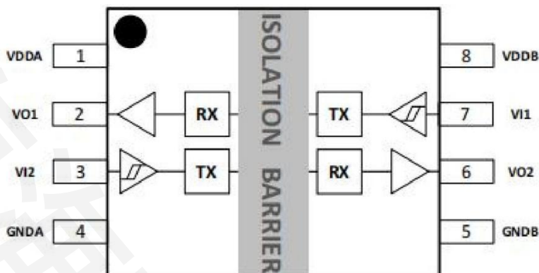
图 1. ISO7221ADR-HX/ISO7221BDR-HX/ISO7221CDR-HX SOP08(窄体)封装顶部视图
