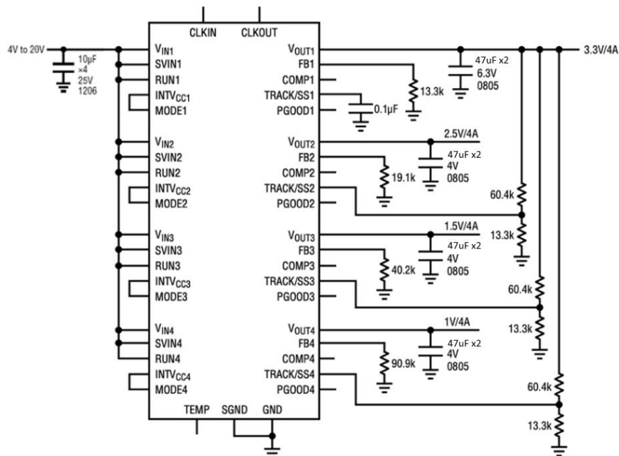
图 19: 具有跟踪功能的 4V 至 20V 输入，四通道 1.0V，1.5V，2.5V 和 3.3V 输出
