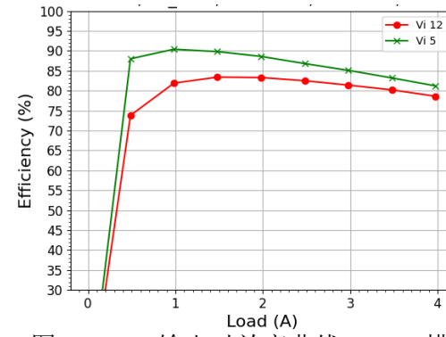
图 3: 1.2V 输出时效率曲线，CCM 模式
