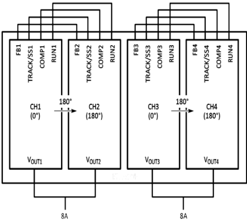
图 15: 2+2 通道并联概念示意图
