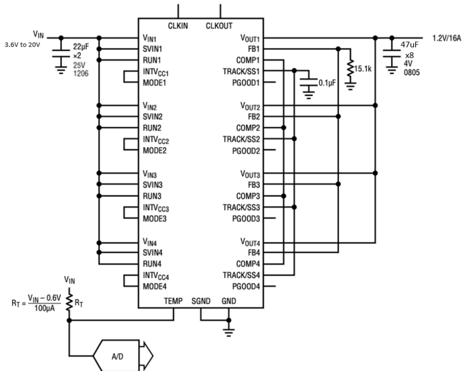
图 20: 单通道 3.6V 至 20V 输入，4 相，1.2V 输出，16A 设计，带温度监控
