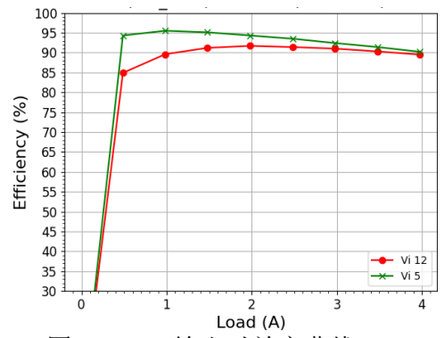
图 4: 3.3V 输出时效率曲线，DCM 模式
