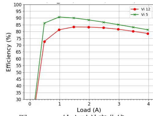
图 5: 1.2V 输出时效率曲线，DCM 模式
