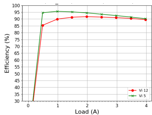
图 2: 3.3V 输出时效率曲线，CCM 模式
