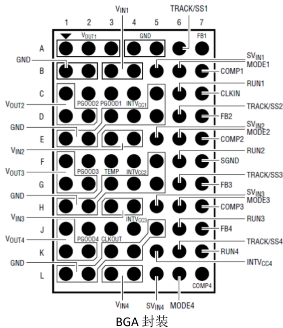
图 1: SPES4644OT 封装顶视图
