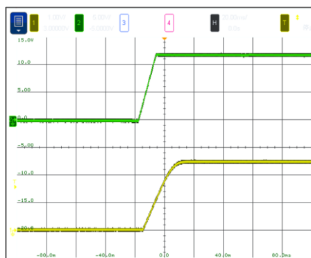
12Vin, 2.5Vout, 0A
