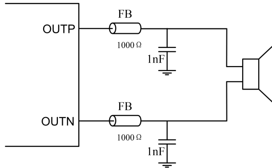
输出端加磁珠应用图
