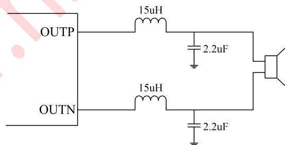
负载为 4Ω, 转折频率为 27kHz 的 LC 输出滤波器
