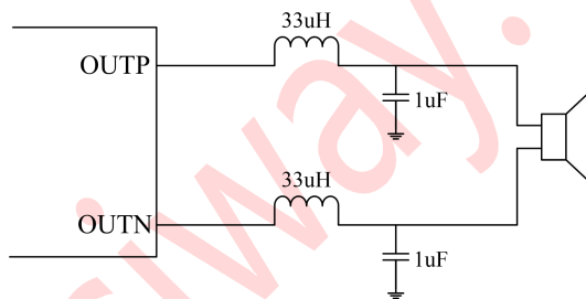
负载为 8Ω, 转折频率为 27kHz 的 LC 输出滤波器
