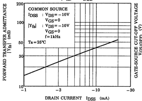
|Y_{fs}| - I_{DSS}
