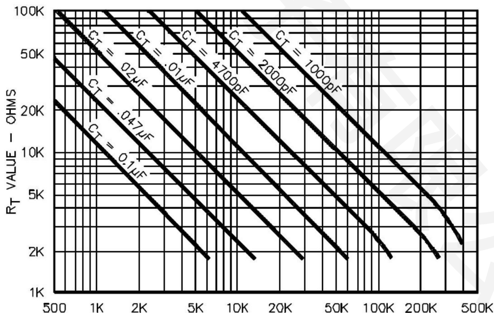
振荡频率与 R_t 、 C_t 关系
