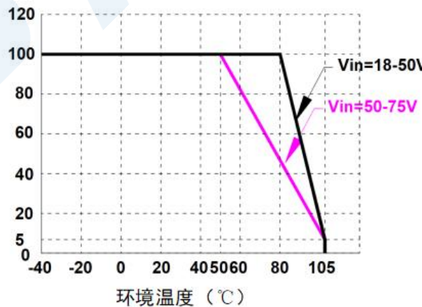
温度降额曲线图（URB4812/24YMD-40WR3）图 2-2
