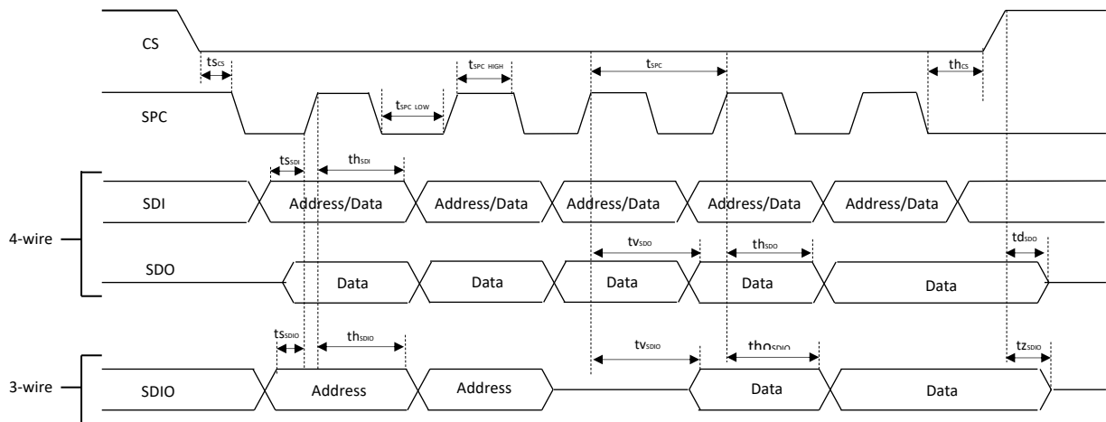
SPI : Mode 3
