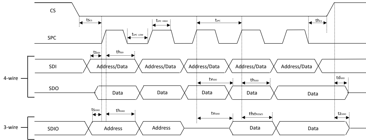
SPI : Mode 0
