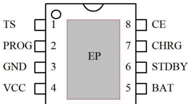
TP4056H ESOP-8
