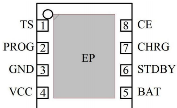
TP4056H DFN8-3*3
