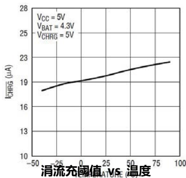
CHRG 引脚电流 vs 温度 (弱下拉)
