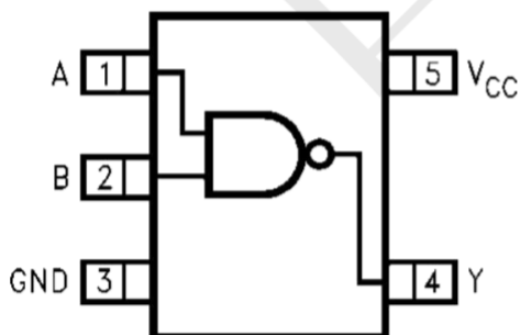
SOT353
