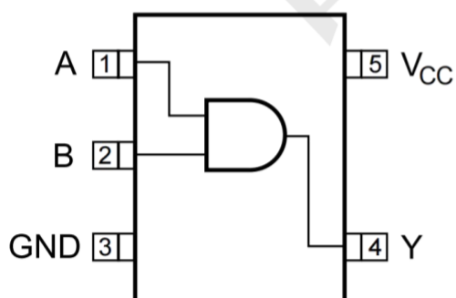
SOT353
