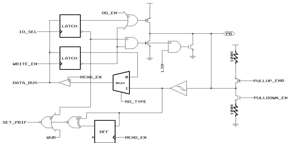
图 7 PB1 引脚结构框图
