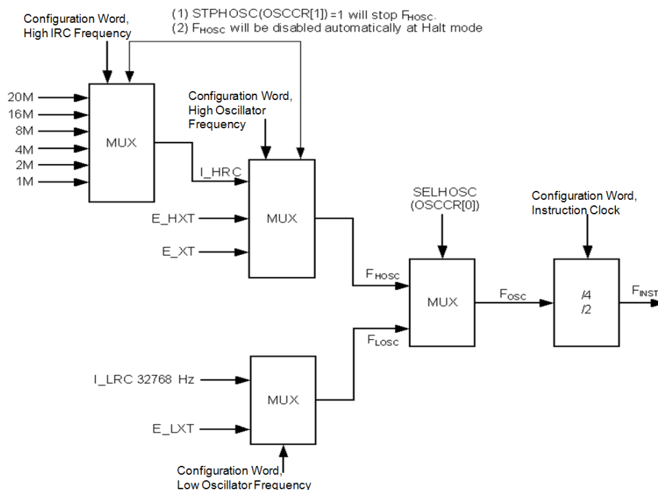
图 22 NY8A053E振荡配置结构图
