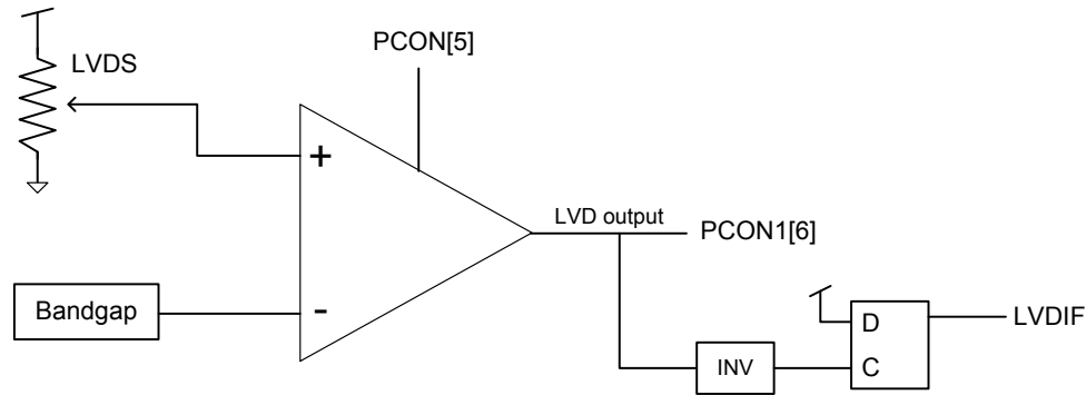
图 19 LVD结构框图
