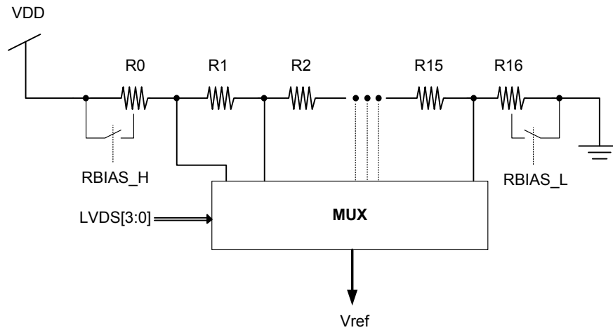
图 21 Vref 结构框图
