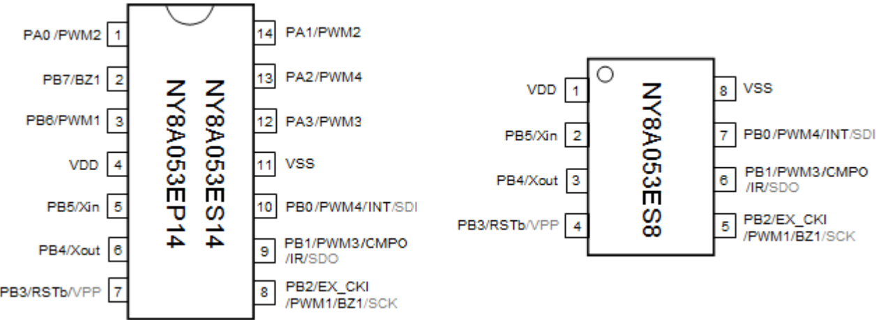
图 1 封装引脚图
