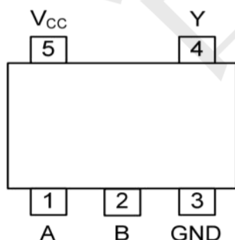
SOT353
