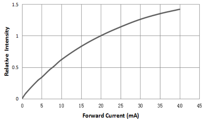
相对光强与电流特性曲线
