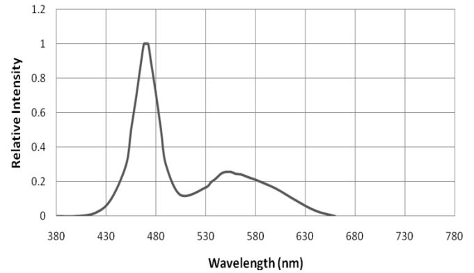
光谱分布特性曲线
