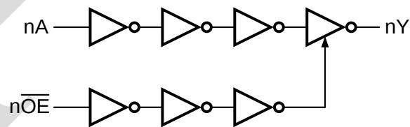
图 3 逻辑框图
