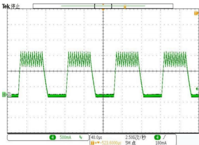
Fdim=10KHz Duty=50%
