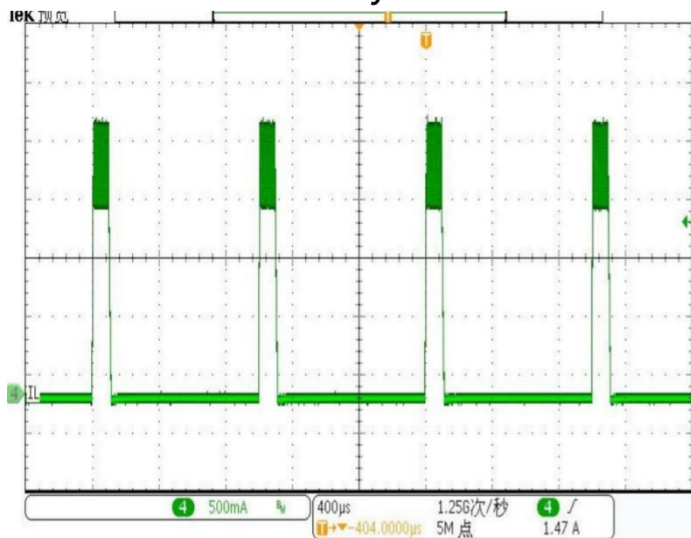
Fdim=1KHz Duty=10%
