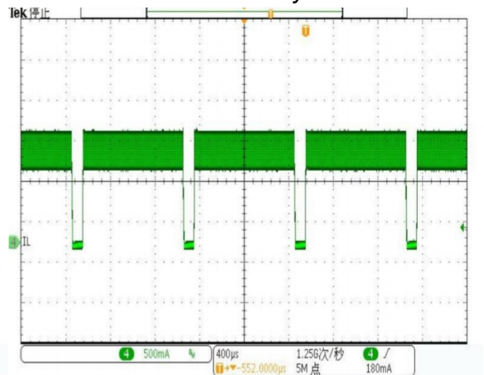
Fdim=1KHz Duty=90%
