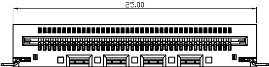
40PIN
