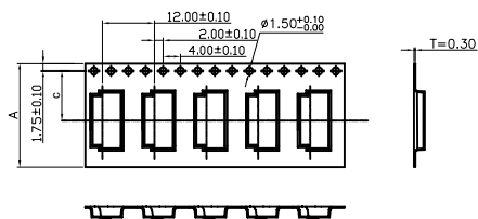
4~23PIN REEL
